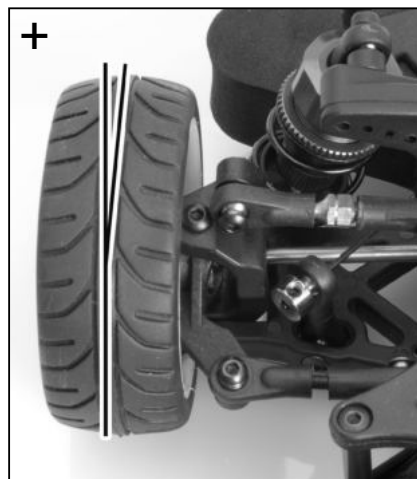
+ Vorspur Toe In Pinçage Convergencia positiva
