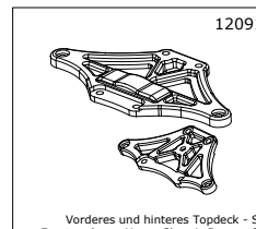
120913 Vorderes und hinteres Topdeck - S10 Front and rear Upper Chassis Brace - S10
