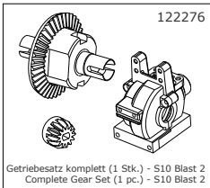
122276 Getriebebesatz komplett (1 Stk.) - S10 Blast 2 Complete Gear Set (1 pc.) - S10 Blast 2
