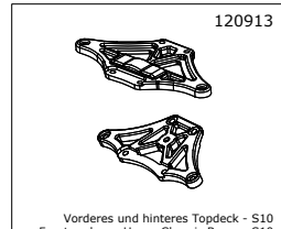
Vorderes und hinteres Topdeck - S10 Front and rear Upper Chassis Brace - S10
