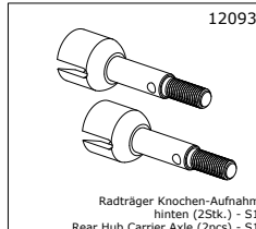
120935 Radträger Knochen-Aufnahme hinten (2Stk.) - S10 Rear Hub Carrier Axle (2pcs) - S10
