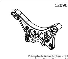
Dämpferbrücke hinten - S10 Rear Shock Tower - S10
