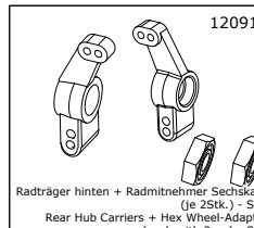
120910 Radträger hinten + Radmitnehmer Sechskant (je 2Stk.) - S10 Rear Hub Carriers + Hex Wheel-Adapter (each with 2pcs) - S10
